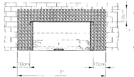
Stenový trezor bez zadnej pancierovej steny
