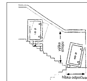
Obr.: č. 6: schody otočené o 180 stupňov s odpočívadlom
